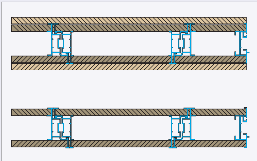
Módulos de Puerta Door Modules
