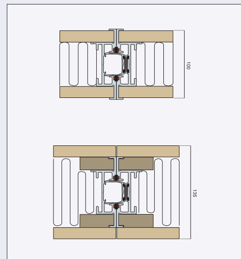
Unión Tipo entre Módulos Module Union Types
