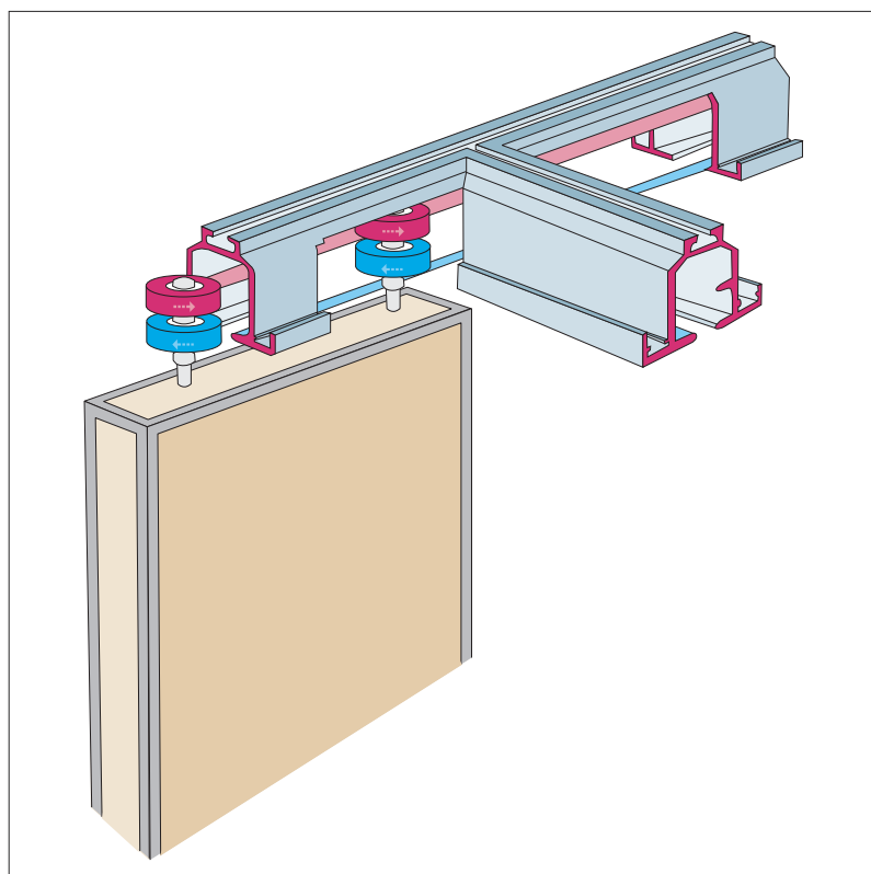
Detalle de poleas e intersección en la guía. Detail of pulleys and intersection in the guide.
